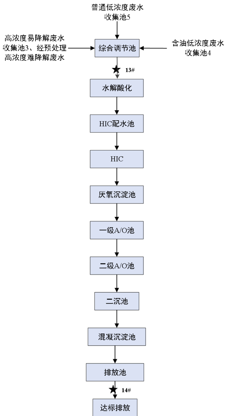
图 7.1-5 8#普通低浓度废水处理工艺流程图
