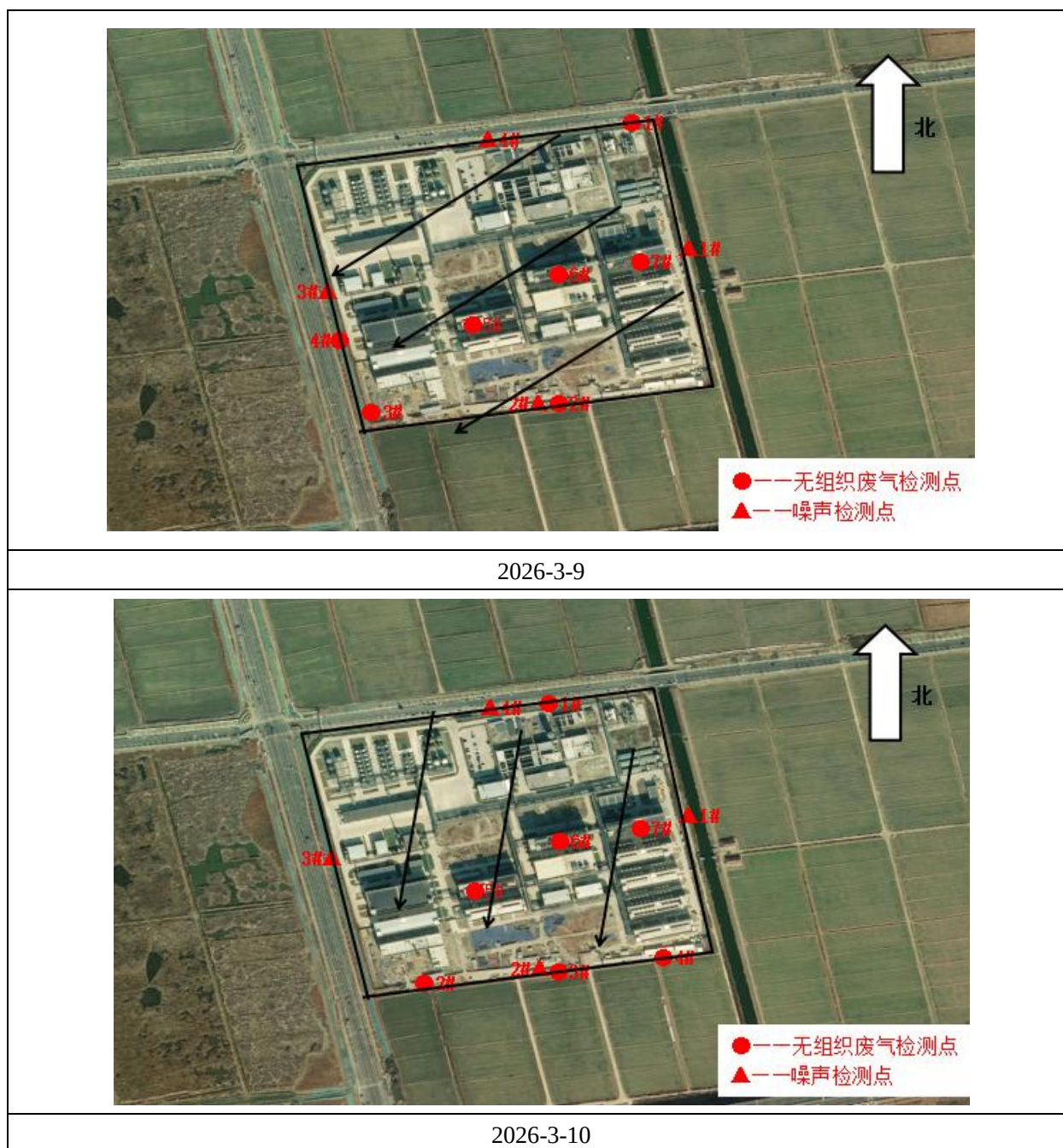
图 7.1-7 无组织废气及噪声监测布点图
