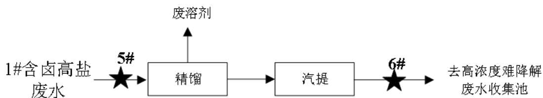
图 7.1-1 1#含卤高盐废水预处理工艺流程图
