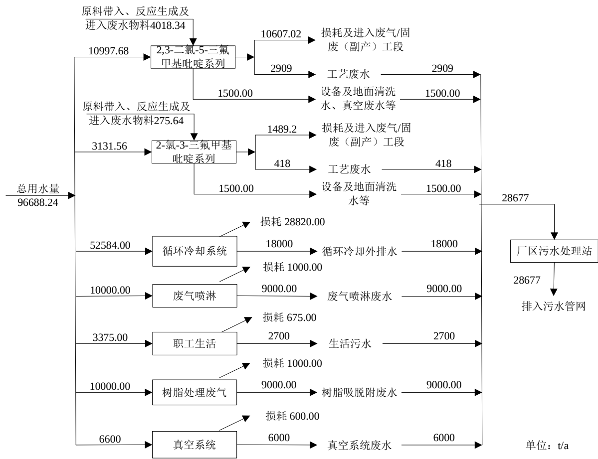
图 3.5-1 项目水平衡图
