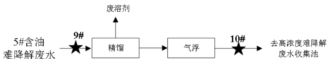
图 7.1-3 5#含油难降解废水预处理工艺流程图
