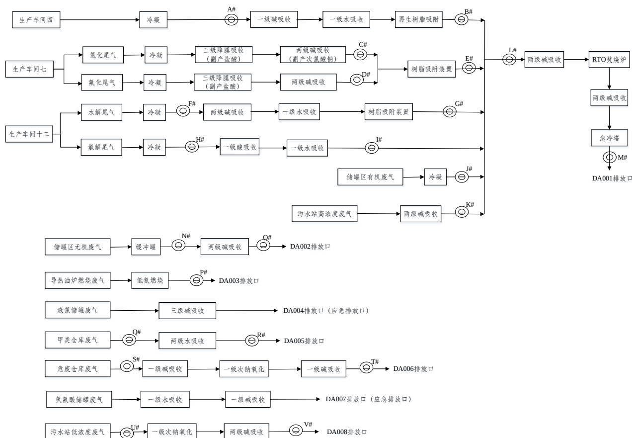
图 7.1-6 有组织废气监测布点图
