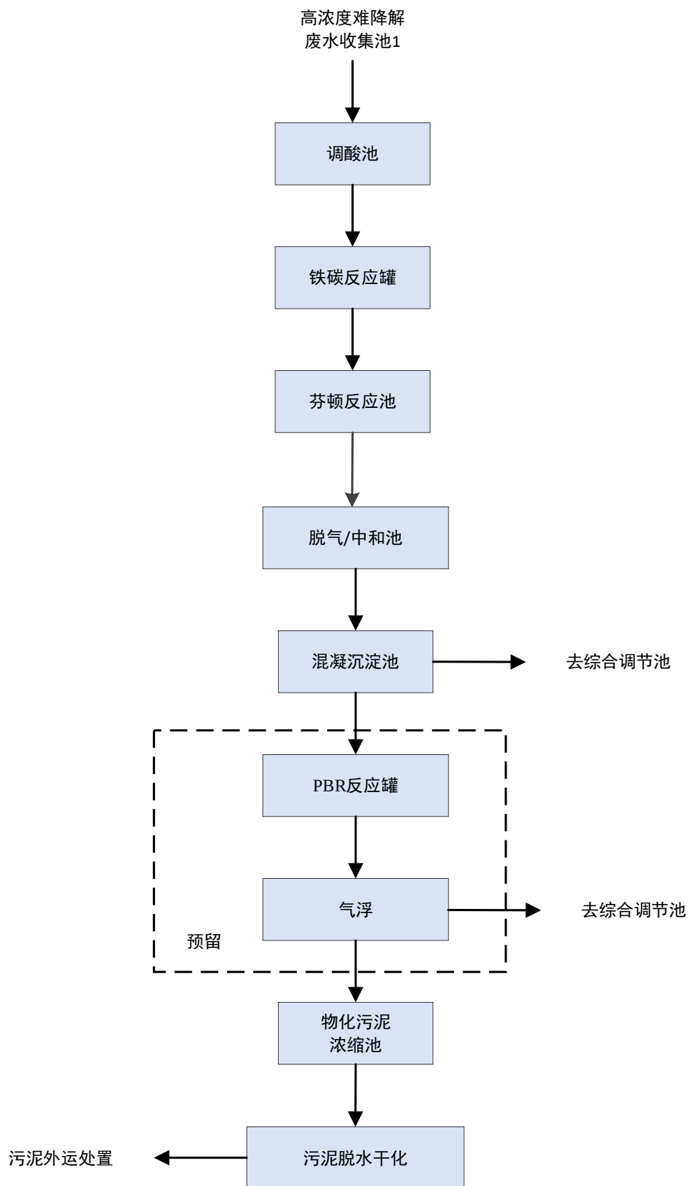
图 4.1-4 高浓度难降解废水预处理工艺流程图
