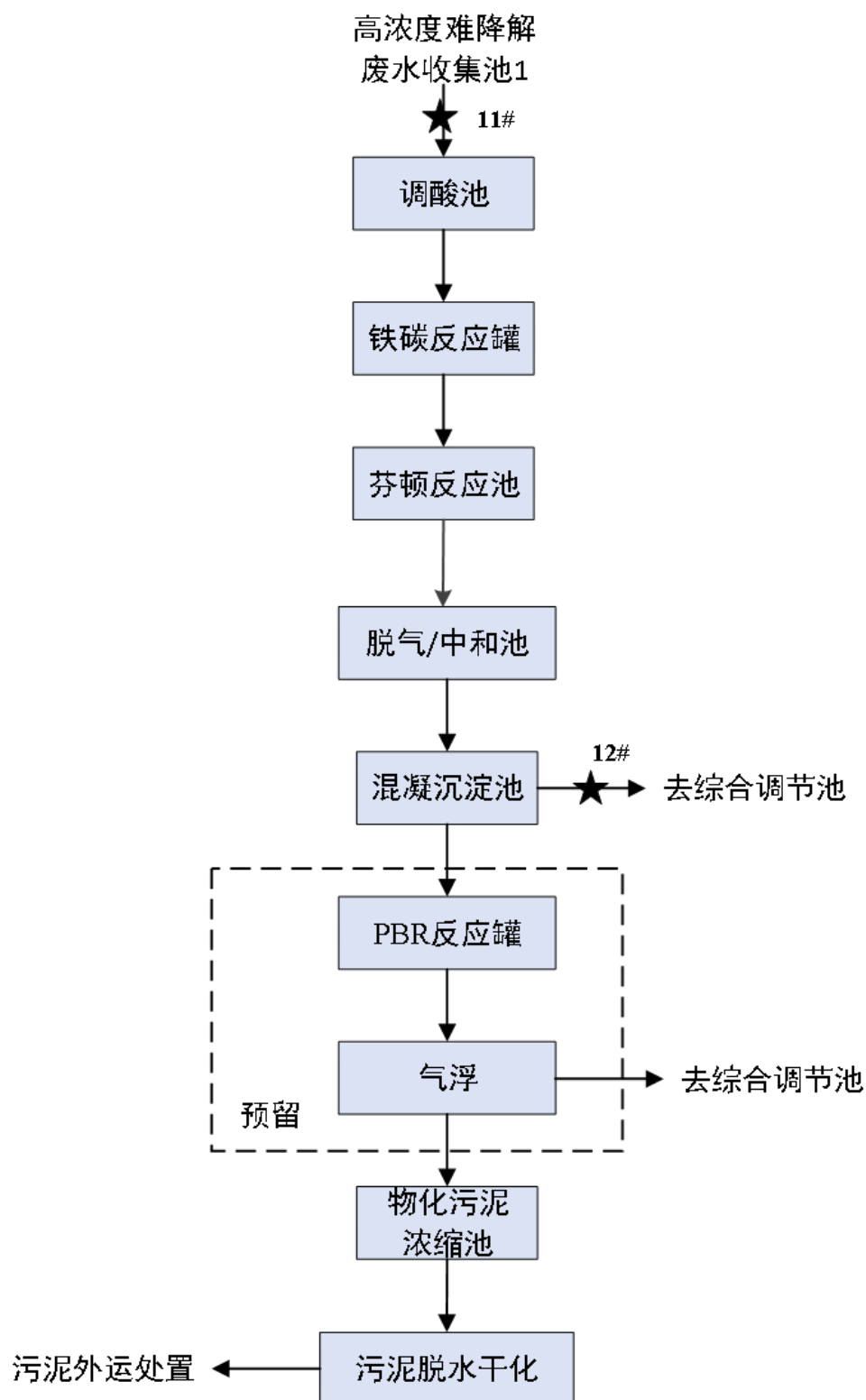
图 7.1-4 3#高浓度难降解废水预处理工艺流程图
