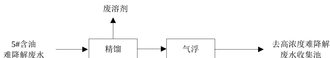
图 4.1-3 5#含油难降解废水预处理工艺流程图
