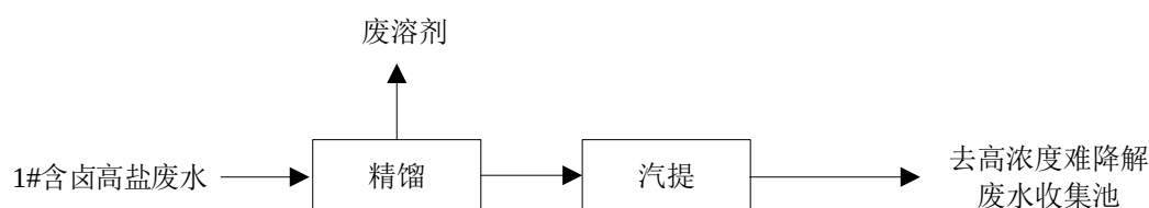
图 4.1-1 1#含卤高盐废水预处理工艺流程图
