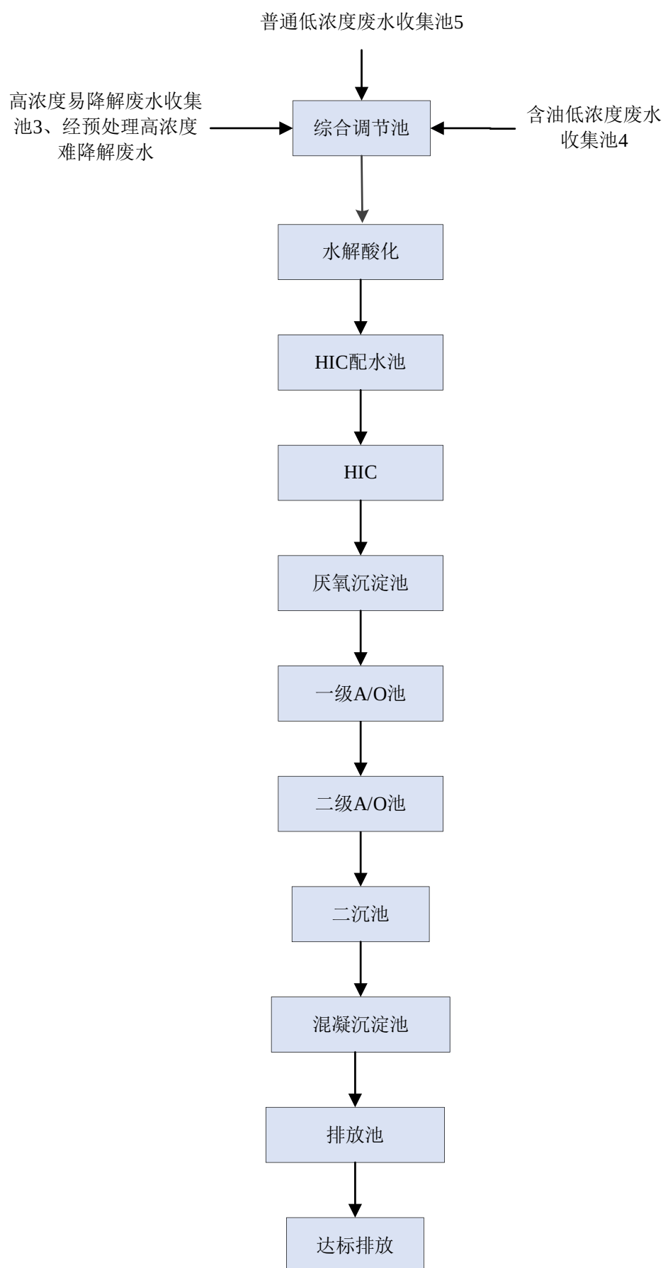
图 4.1-5 综合废水处理处理工艺流程
