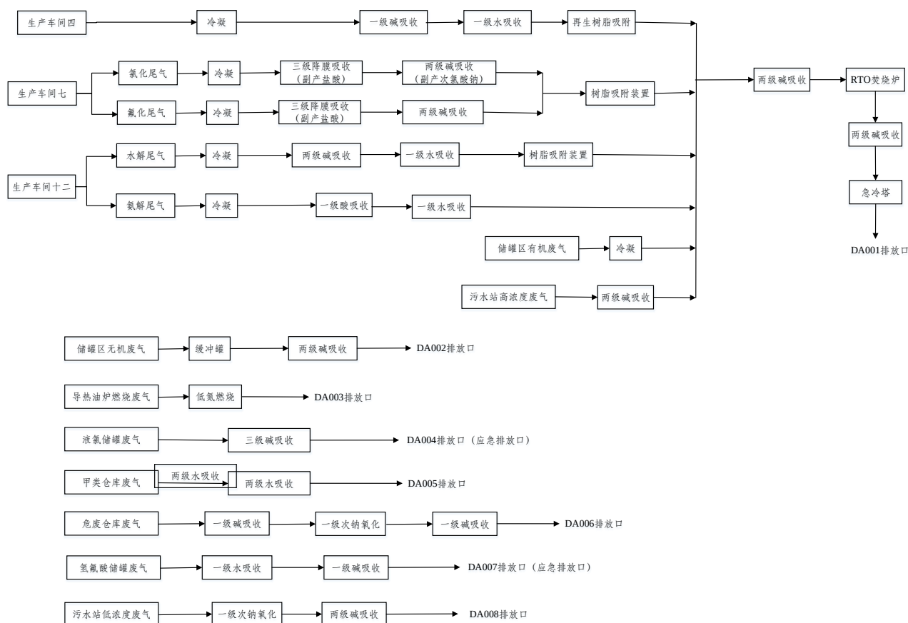
图 4.1-7 项目本期建设内容及同期验收项目实施后废气（全厂）处理工艺流程
