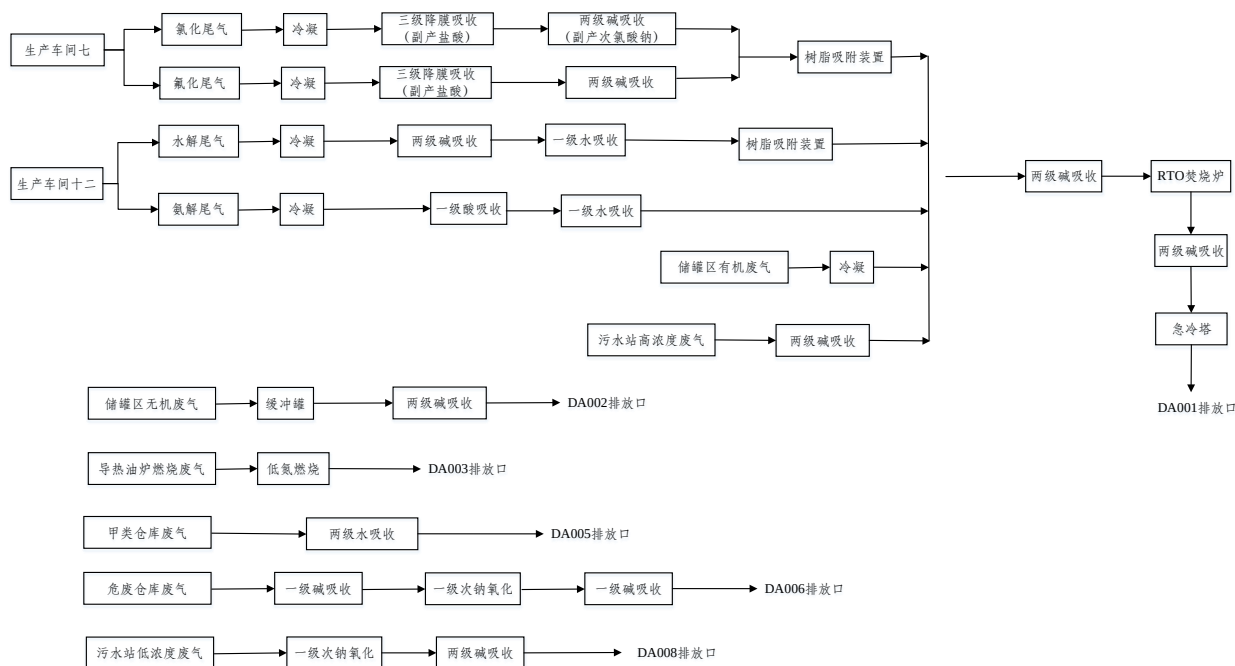
图 4.1-6 项目本期建设内容废气处理工艺流程
